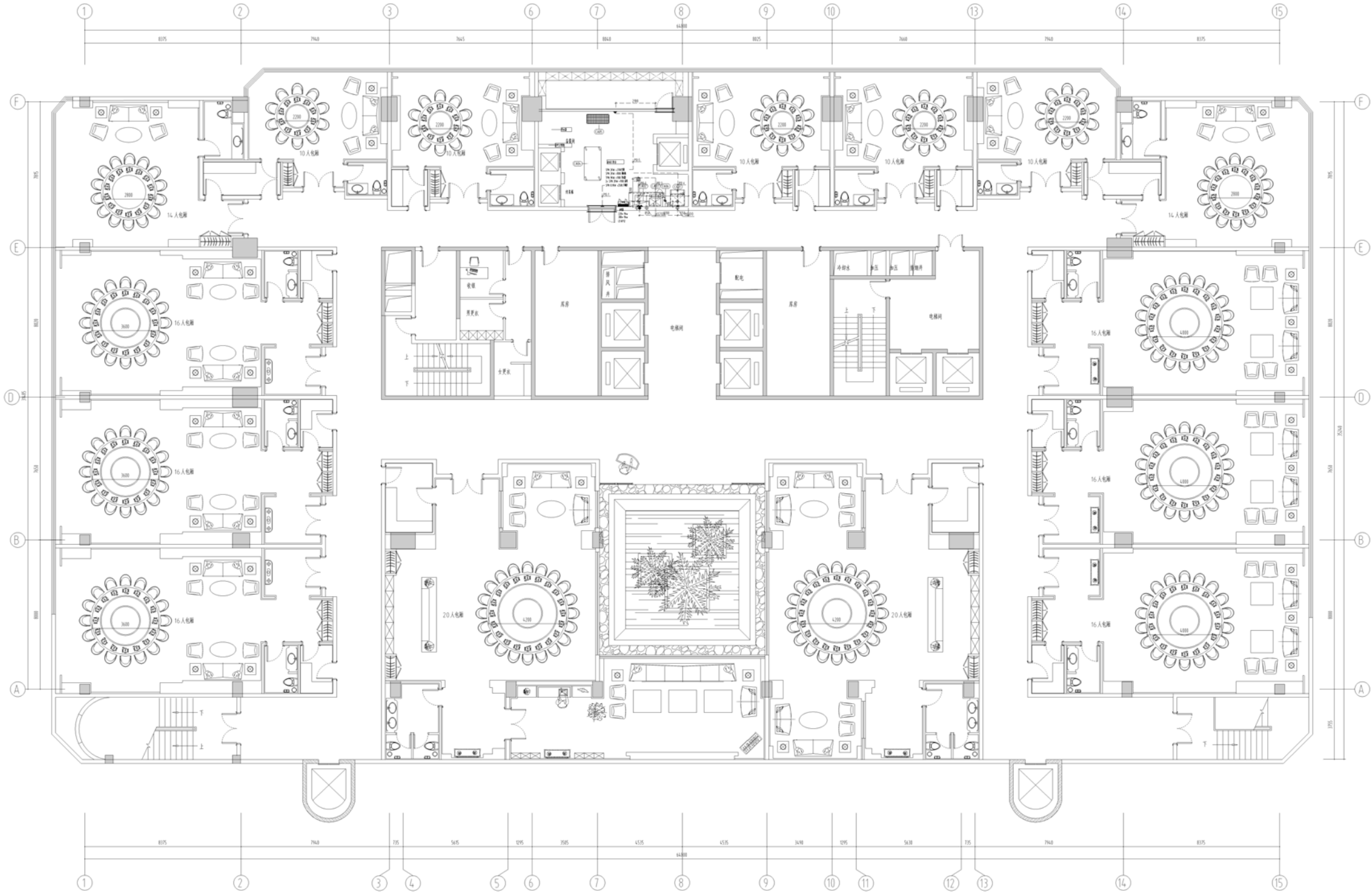
三楼平面布置图(部分房与实际现场有些不同)
